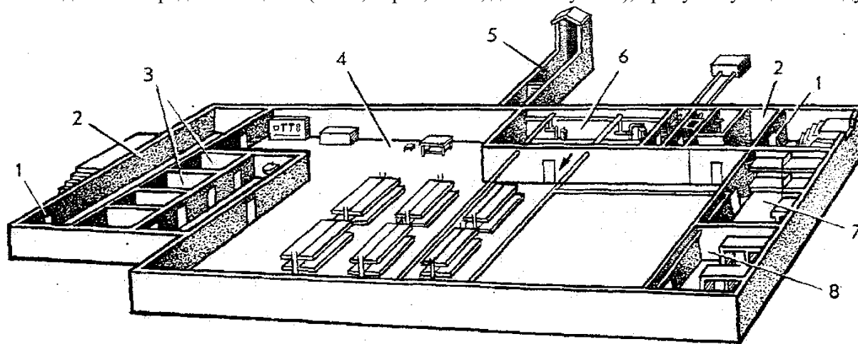
Рисунок 2.1 – План убежища
